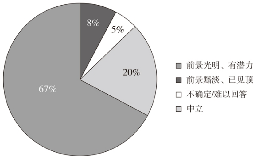
图3 中国经济发展前景全球民意调查
