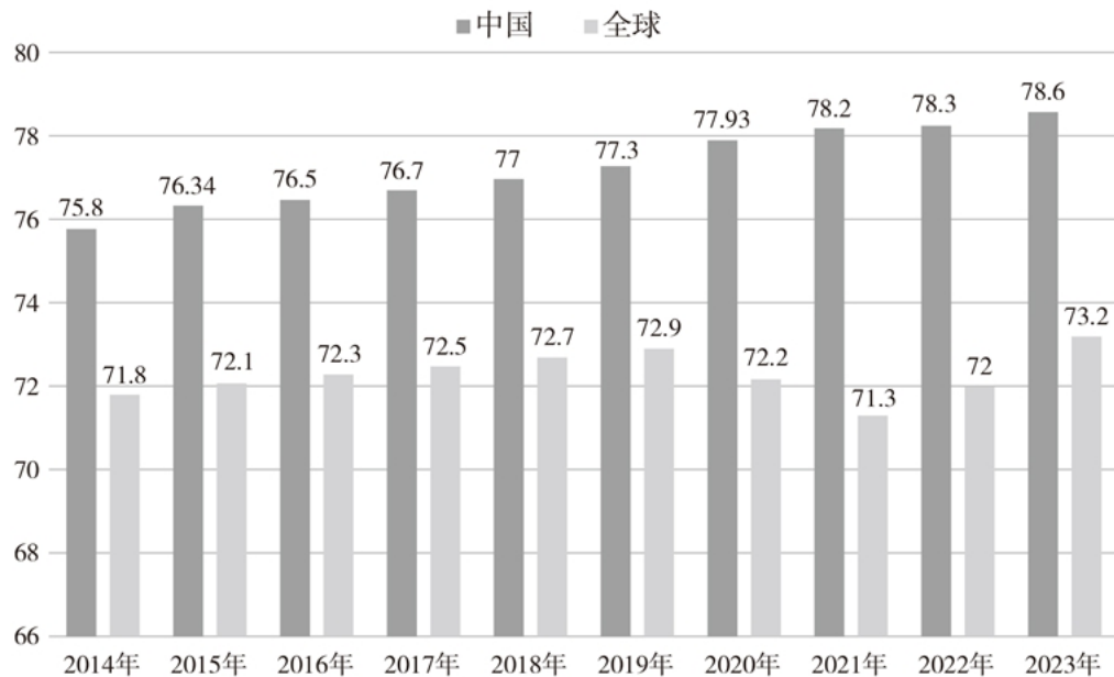
图 1 2014 年至 2023 年中国和全球人均预期寿命比较(岁)
