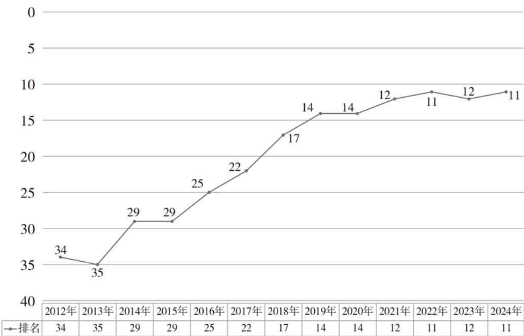
图 2 2012 年至 2024 年中国的全球创新指数排名
